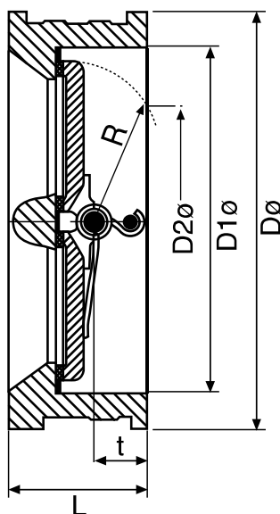
311 Dimensions Table
